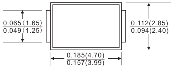
DO-214AC(SMA J-Bend)
