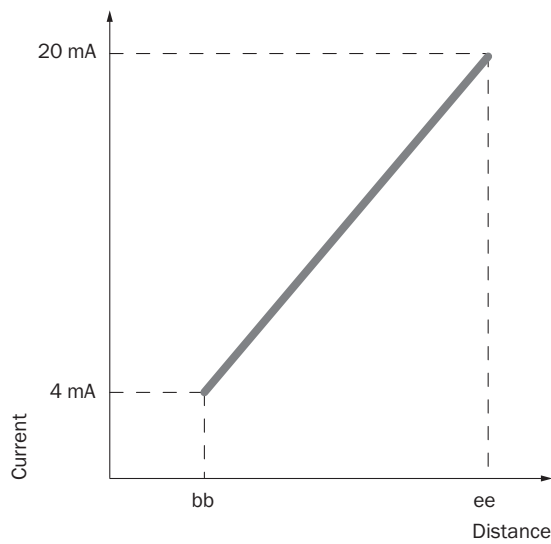
ee > bb
