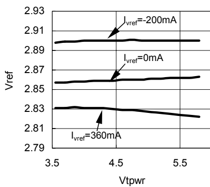
Vref - Vtpwr@T=24°C
