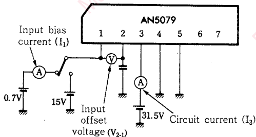
Test Circuit 3 ( I_1 , V_{2-1} , I_3 )
