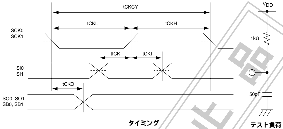
図6 シリアル入出力テスト条件
