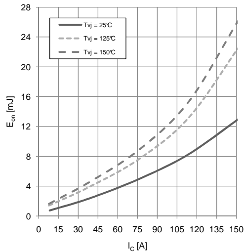
Einschaltverluste IGBT-Wechselr. (typisch) turn-on switching losses IGBT inverter (typical) E_{on} = f(I_C) V_{ge} = \pm 15V, R_{gon} = 2.2\Omega, V_{ce} = 600V
