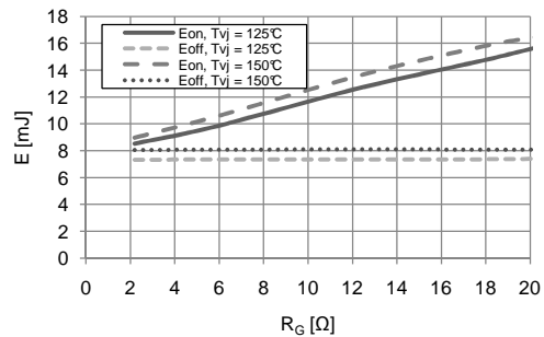
Schaltverluste IGBT-Wechselr. (typisch) switching losses IGBT inverter (typical) E_{on} = f(R_G), E_{off} = f(R_G) V_{GE} = \pm 15V, I_C = 75A
