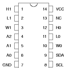
DS1803E 14-PIN TSSOP (173 MIL)
