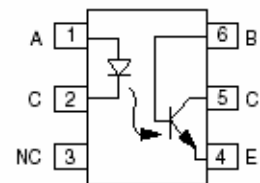
CNY17-X
