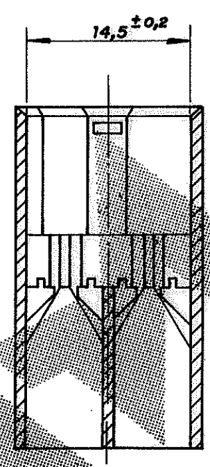
SECÇÃO A:A
