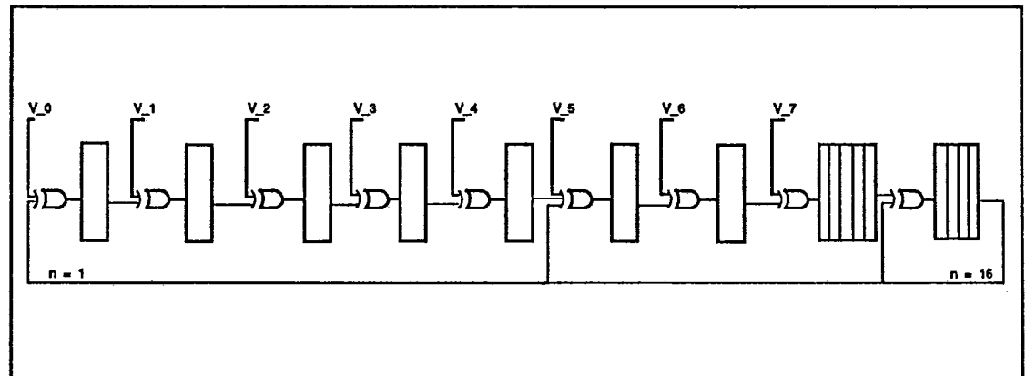
FIGURE B-1. LINEAR FEEDBACK SHIFT REGISTER
