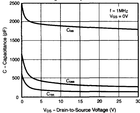
Fig. 8 – Capacitance
