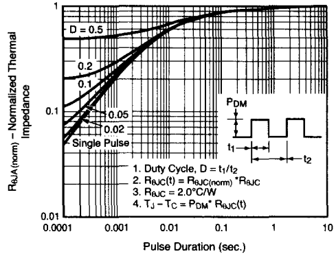
Fig. 11 – Transient Thermal Impedance
