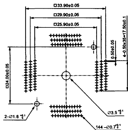
QFP IC234-1444-016 (144 Pins)
