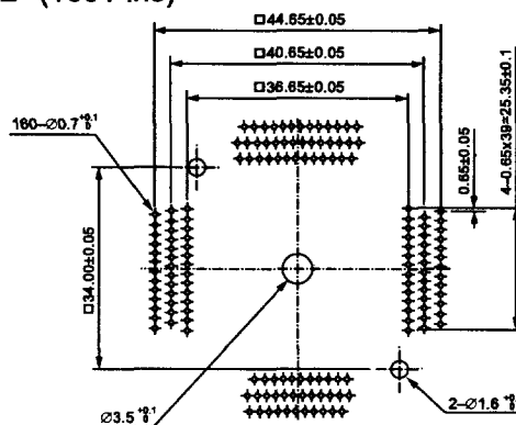
QFP IC234-1764-005 (176 Pins)
