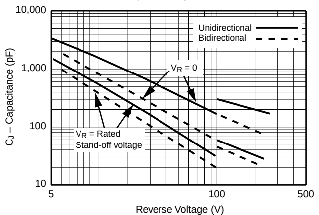
Fig. 6 – Capacitance
