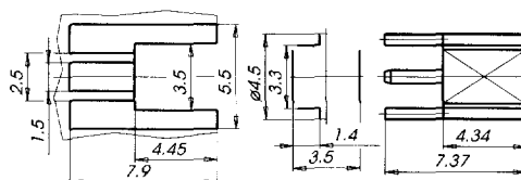
SMT - Lötflächen Solderpad Layout
