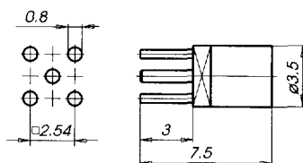
Montagebohrungen Mounting Detail
