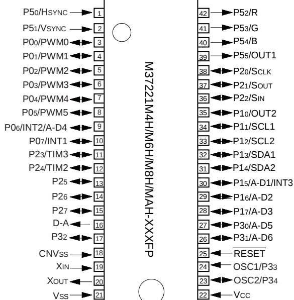
Outline 42P2R-A/E
