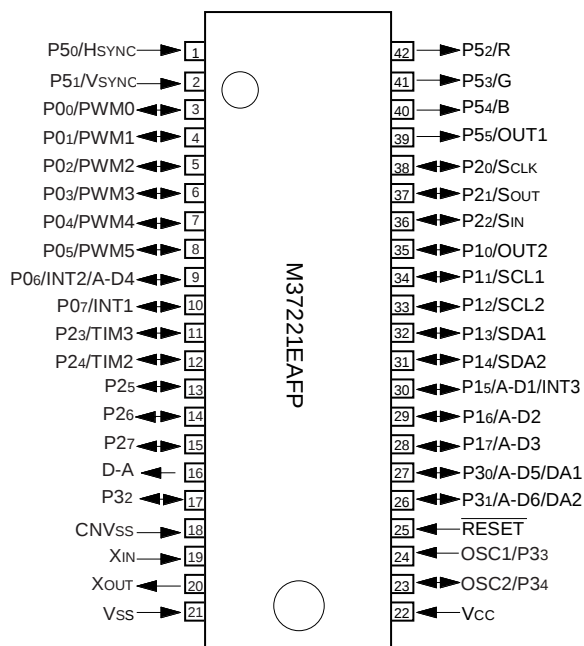
Outline 42P2R-A/E
