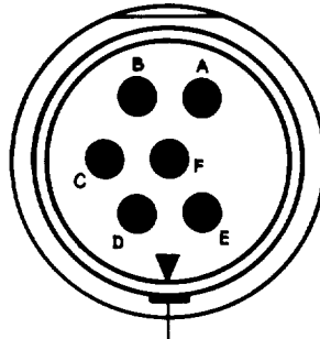
Datum keyway/key
