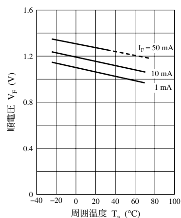
V_F - T_a
