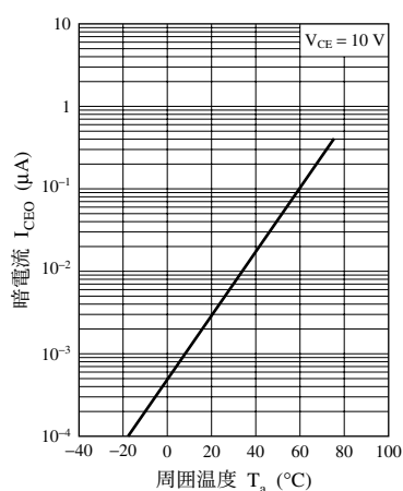
I_{CEO} - T_a
