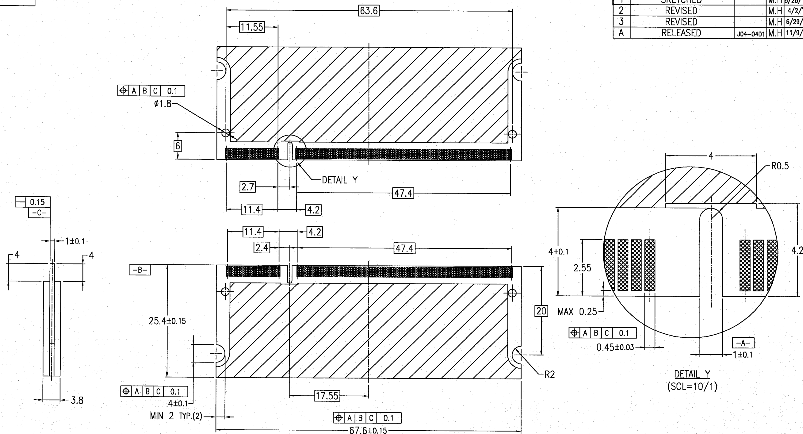
RECOMMENDED MODULE P.C.B LAYOUT
