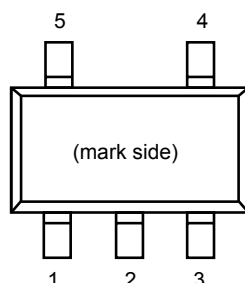
SOT-23-5
