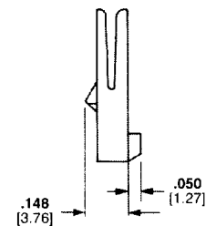
Detent
