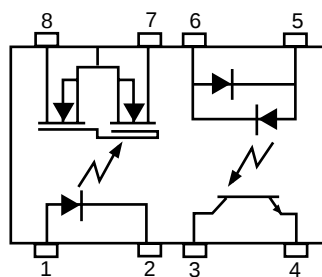
AC Hybrid: Optocoupler plus SSR
