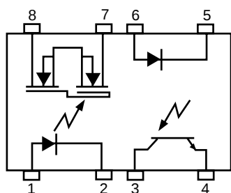
DC Hybrid: Optocoupler plus SSR
