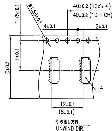
図2-1. エンボステープ詳細 (P/N 10013057-17120_ELF~ 10013057-45120_ELF)
