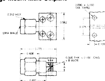
Edge Mount Male Stripline
