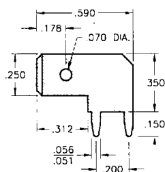
.250 TAB
