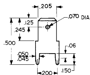
.205 TAB
