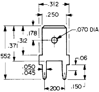
.250 TAB
