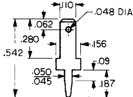
.110 TAB
