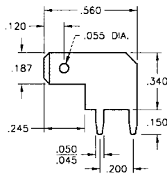
.187 TAB
