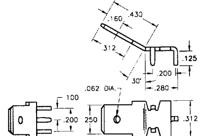
.250 TAB
