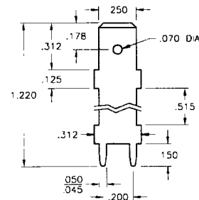
.250 TAB
