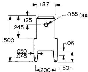
.187 TAB
