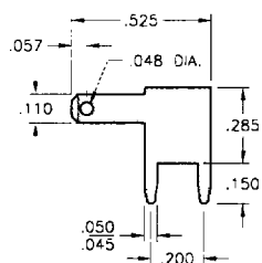
.110 TAB
