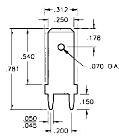
.250 TAB
