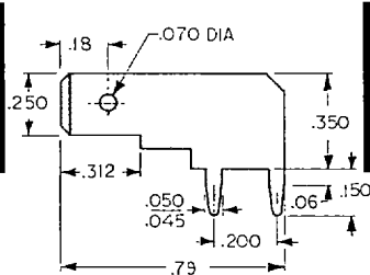
.250 TAB
