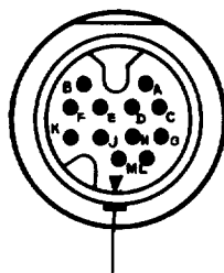
Datum keyway/key
