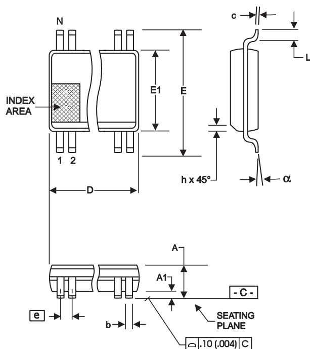
300 mil SSOP
