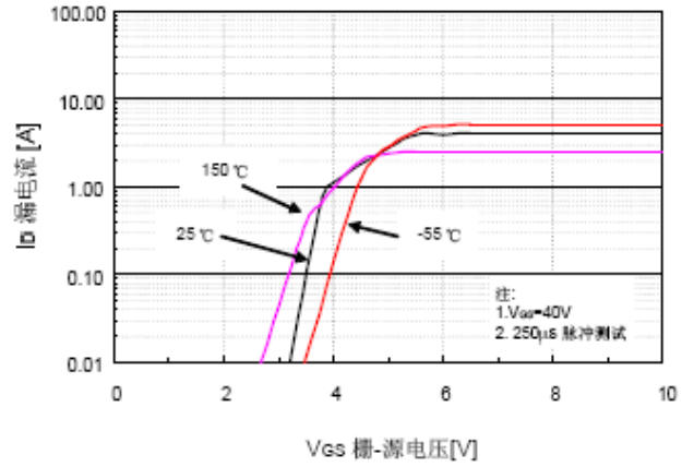
图2、传输特性
