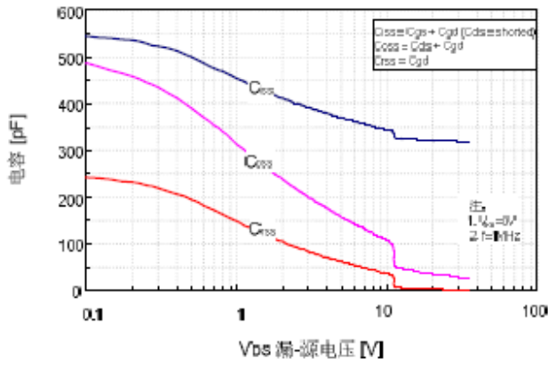
图5、电容特性
