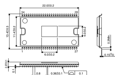
SSOP-A54
