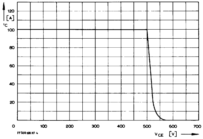
4 Erlaubter Arbeitsbereich in Rückwärtsrichtung. Reverse biased safe operating area. t_{vj} = 125^\circ\text{C} , V_{LF} = V_{LR} = 15\text{ V} , R_G = 51\ \Omega
