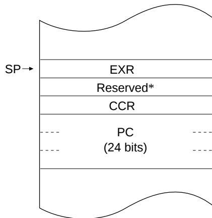
(d) Interrupt control modes 2 & 3
