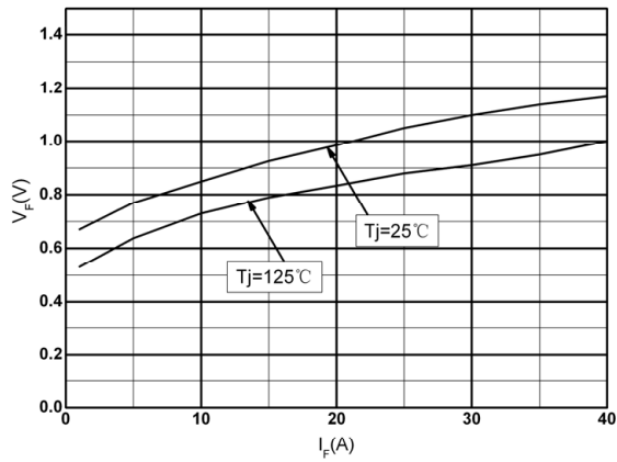
I_F vs V_F
