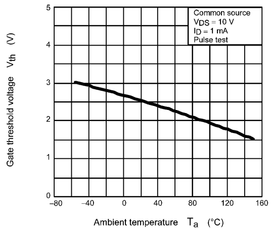
Fig. 8.10 V_{th} - T_a
