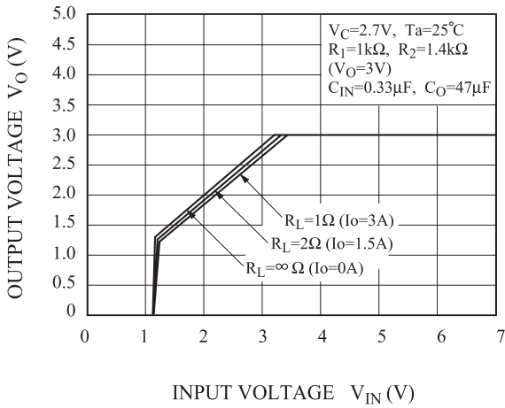
Fig. 6 V_{IN} - V_O
