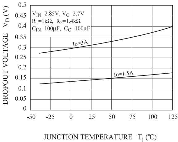
Fig. 8 T_j - V_D
