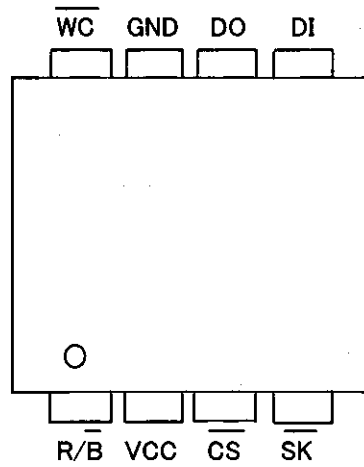
BR9020FV-W: SSOP8 BR9020F-W: SOP8
