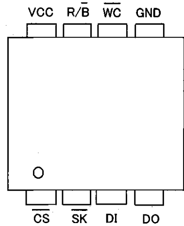
BR9020RFVM-W: MSOP8 BR9020RFV-W: SSOP8
