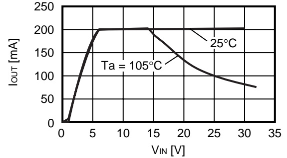
S-1142B50
