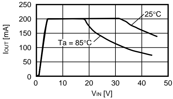
S-1142B33
