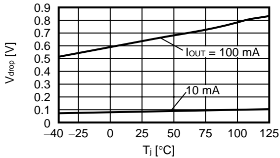
S-1142BC0
