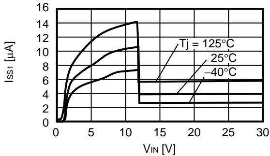
S-1142BC0
