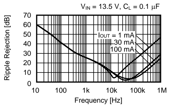
S-1142B50
