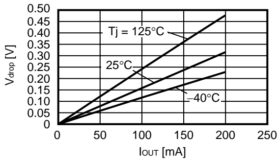
S-1142BC0
