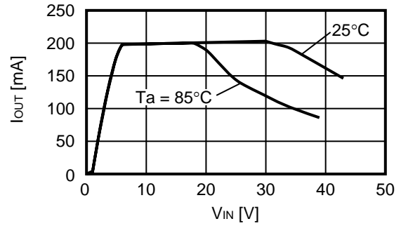
S-1142B50
