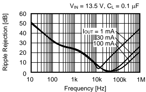
S-1142BC0
