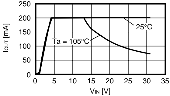
S-1142B33
