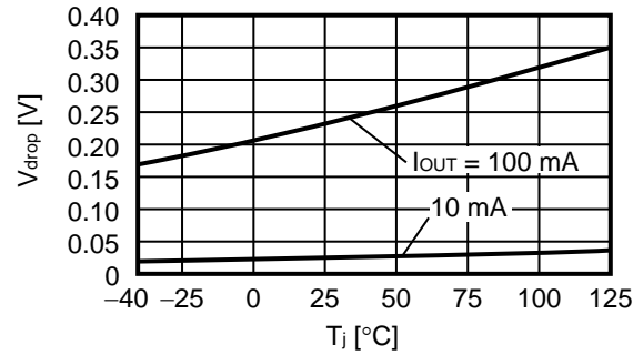
S-1142B50
