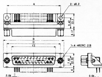
RDBD-25SA-LNA(4-40)
