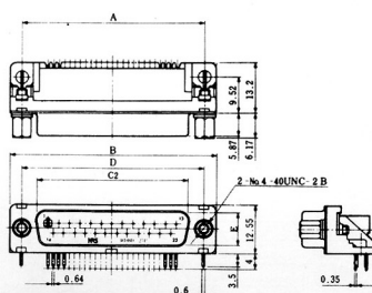
RDBD-25PE-LNA(4-40)
