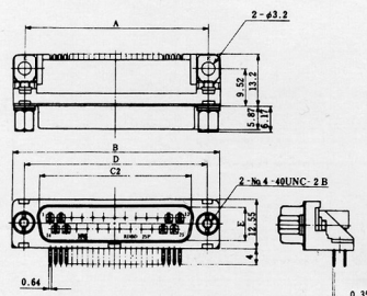
RDBD-25PA-LNA(4-40)
