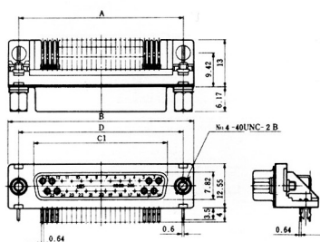
RDBD-25SE-LNA(4-40)
