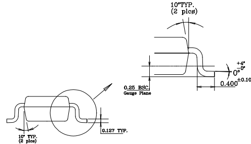
SOT-23-6 (M6)
