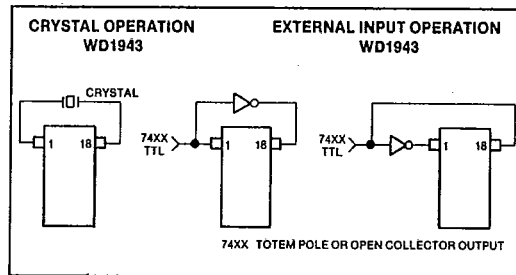
CRYSTAL/CLOCK OPTIONS
