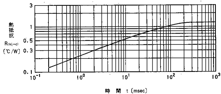
過渡熱抵抗(ツェナーダイオード)特性
