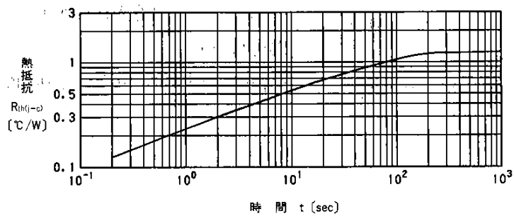
過渡熱抵抗(ダイオード)特性
