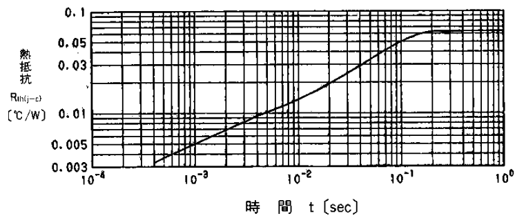
過渡熱抵抗(トランジスタ)特性
