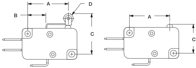
FIG. 1 Lever Roller
