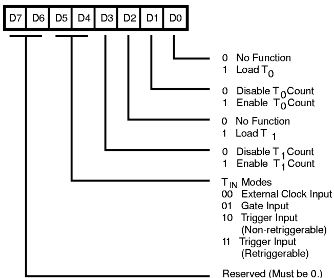
R241 TMR
