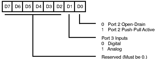
R247 P3M
