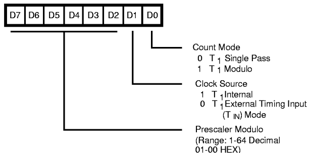
R243 PRE1
