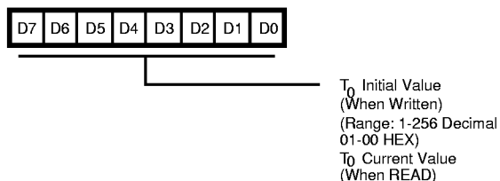
R244 T0
