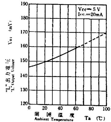
V_{OL} - T_a
