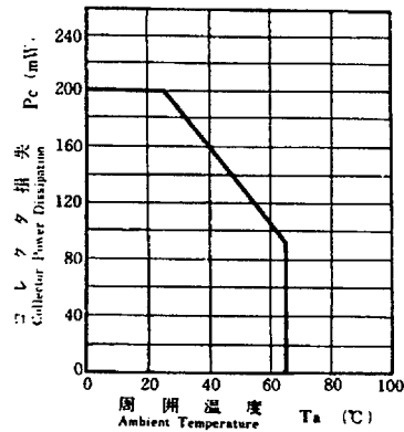
P_c - T_a
