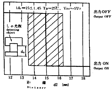
(2) 検知位置特性 Detecting Position Characteristics
