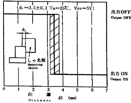
(1) 検知位置特性 Detecting Position Characteristics
