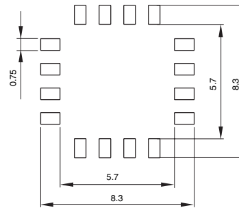
LAND PATTERNS(mm) 推奨ランド寸法
