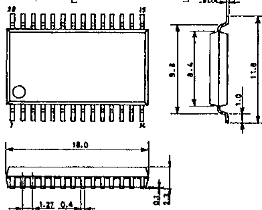
外形図 3187 (unit: mm)
