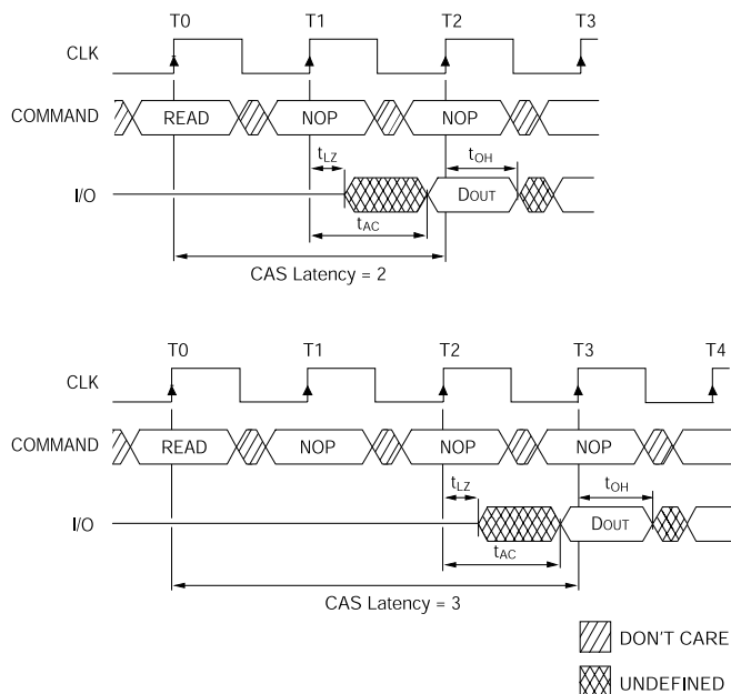
Fig. 4 CAS LATENCY
