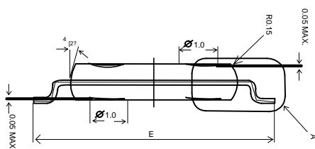
SECTION V-V
