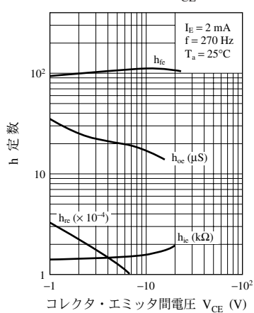
h 定数— V_{CE}
