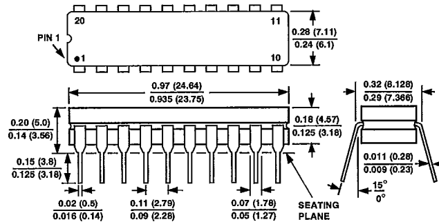
20-Pin Cerdip (R-Suffix)
