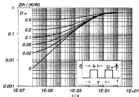
Fig. 4. Transient thermal impedance. Z_{th j-mb} = f(t) ; parameter D = t/T
