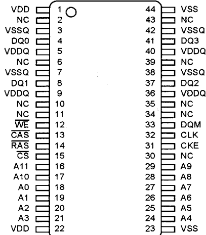
4Mx4 Synchronous DRAM 400mil x 725mil 44pin TSOP-II
